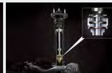
スウィングバルブショックアブソーバー(リヤ)
