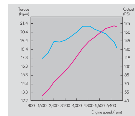
ES 200 引擎動力輸出曲線圖
