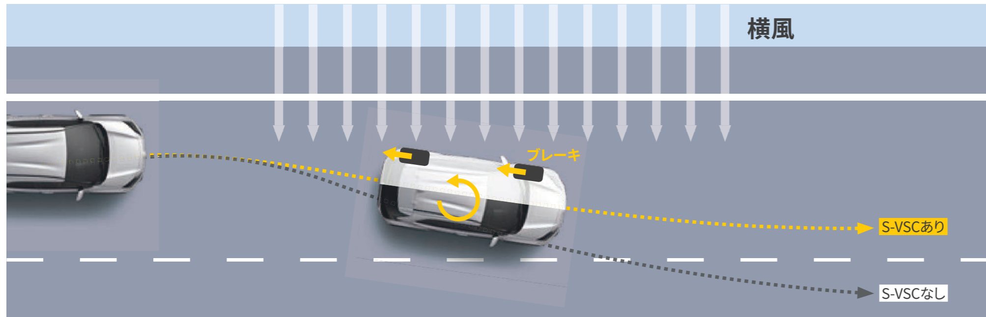
■S-VSC（横風対応制御付）作動イメージ
