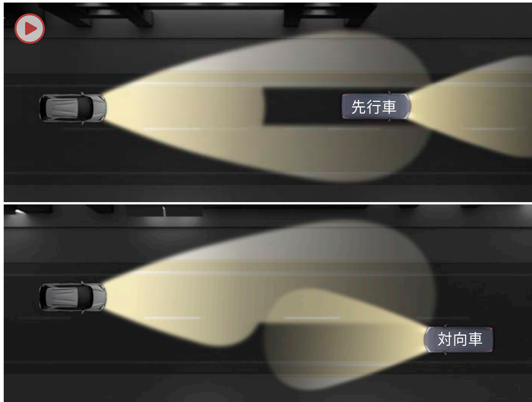
アダプティブハイビームシステム作動イメージ
