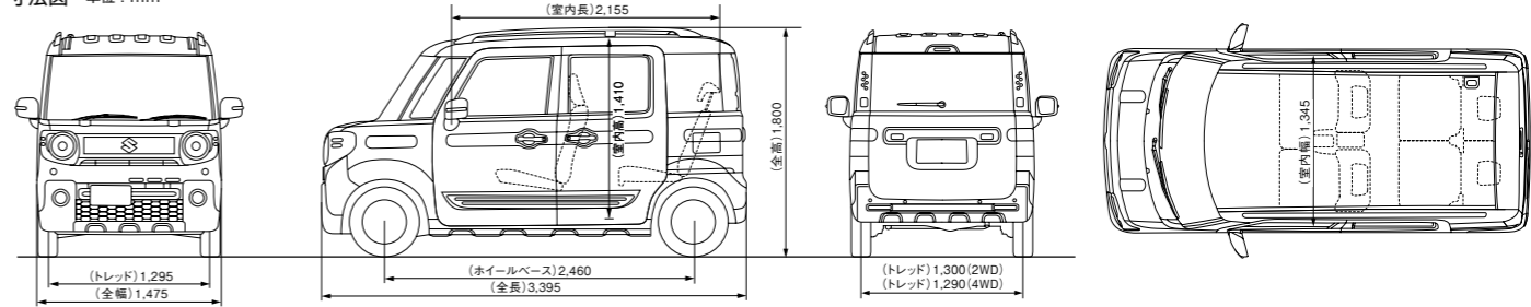
寸法図 単位: mm
