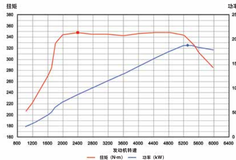
2.0T SIDI直喷涡轮增压发动机功率与扭矩图
