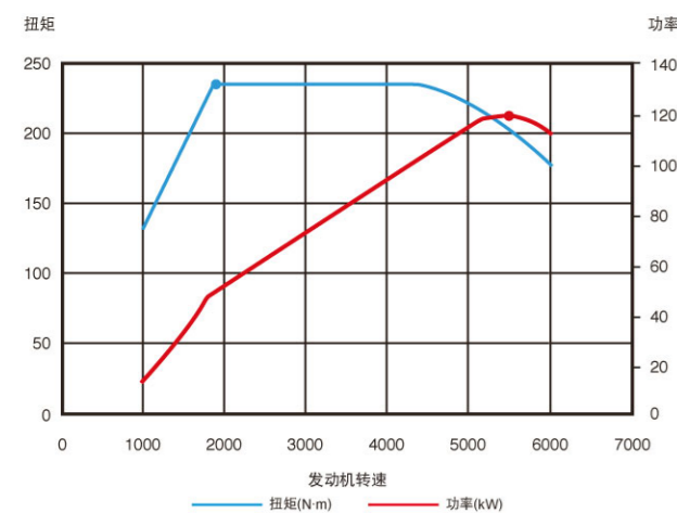
全新一代 1.3T 双喷射涡轮增压发动机功率与扭矩图
