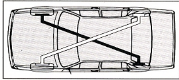
Das Diagonal-Zweikreis-Bremsensystem.
