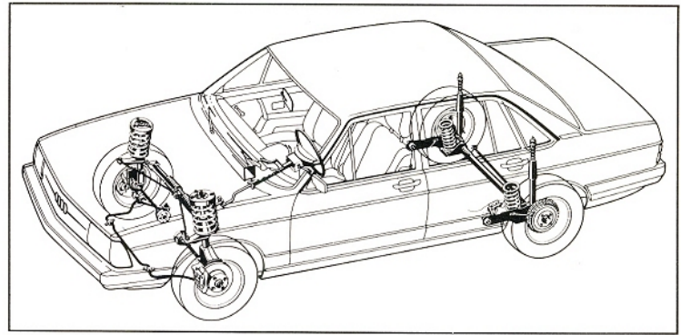
Das aufwendige Komfort-Fahrwerk schluckt selbst große Fahrbahnunebenheiten.
