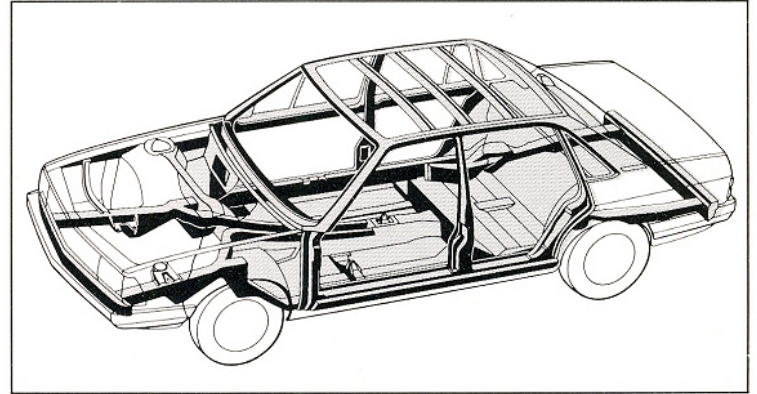
Die moderne Sicherheitskarosserie des Audi 100 CD ist das Ergebnis langjähriger Forschung.
