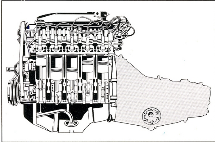
Der 100 kW (136 PS nach DIN)-Fünfzylinder-Motor besticht durch sein besonderes Temperament und seine hohe Laufkultur.
