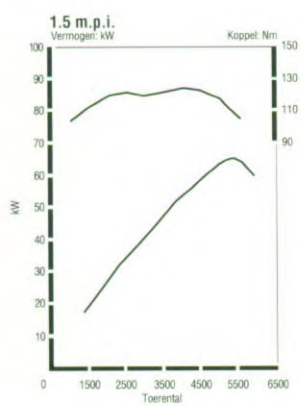
Koppel- en vermogenskromme in Nm en Kw.
