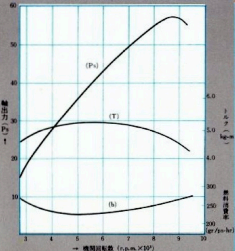
ホンダS 600原動機性能曲線
