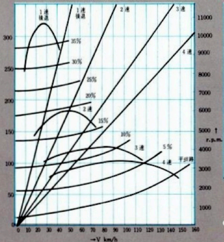
ホンダS 600走行性能曲線
