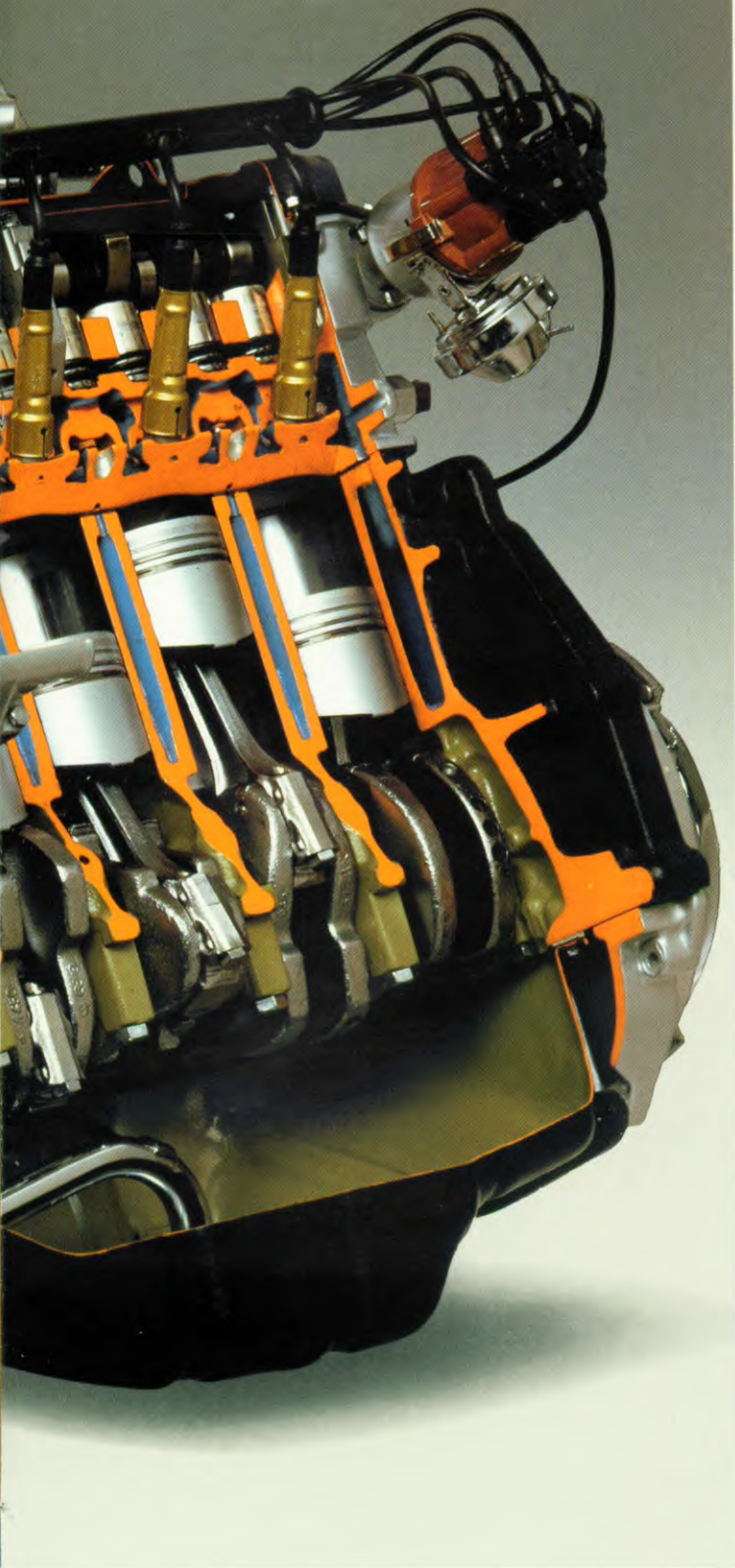
Het injectiesysteem van de vijfcilinder motor
