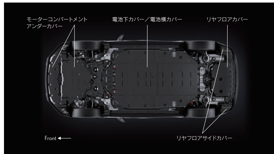
アンダーボディの空力アイテム
